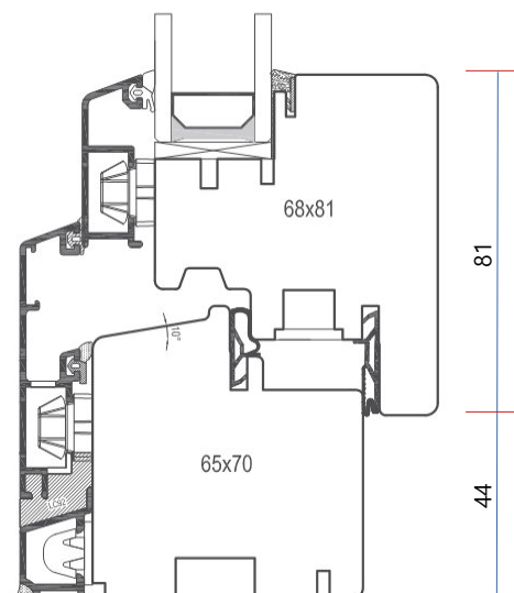
Traverso inf. Finestra
