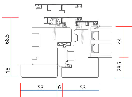
Telaio finestra/portfin.
