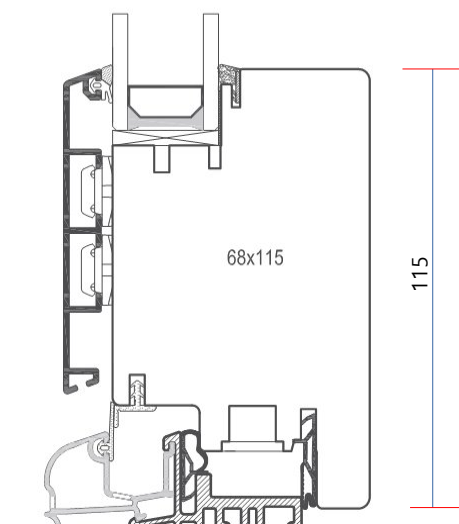
Traverso inf. Porta Fin
