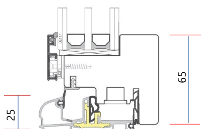
Traverso inferiore portafin.
