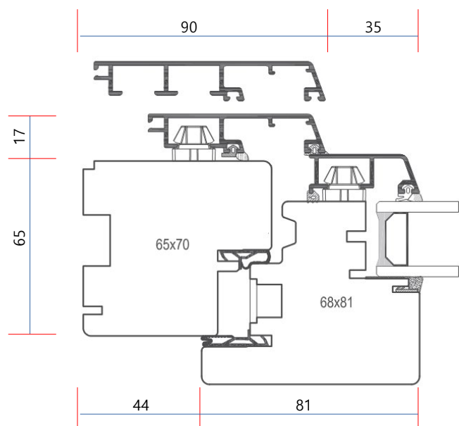
Telaio Fin/Pfin.
