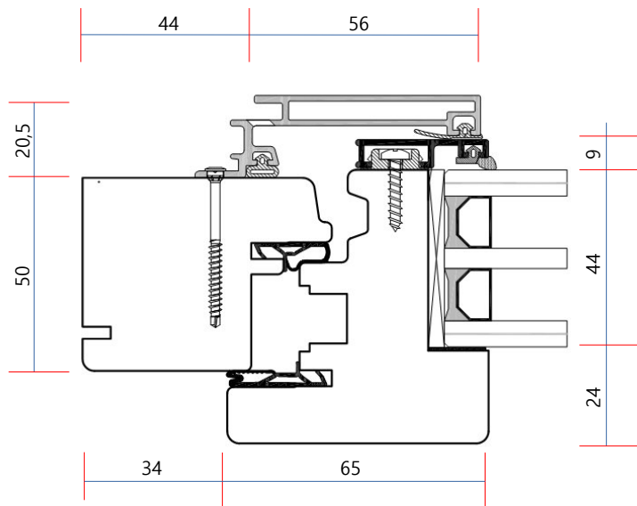
Telaio Fin/Pfin.
