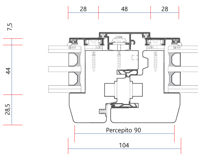
Nodo centrale 2 battenti
