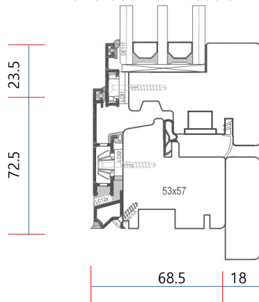
Traverso inf. Finestra
