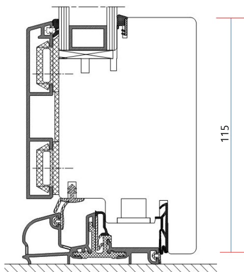
Traverso inf. Portafinestra
