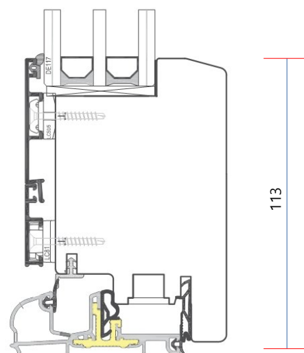
Traverso inf. Portafinestra
