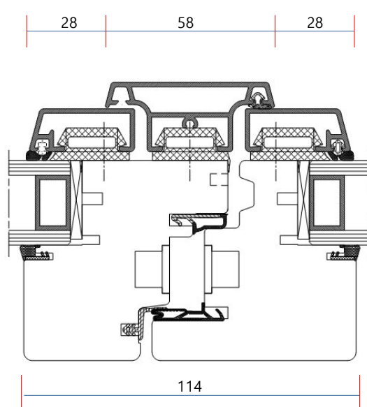
Nodo centrale doppio battente
