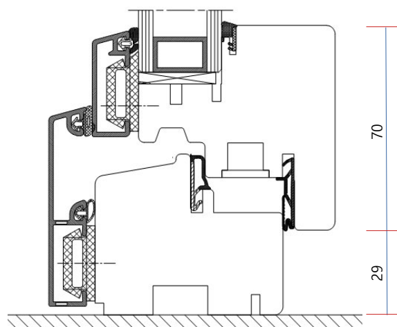
Traverso inf. Finestra
