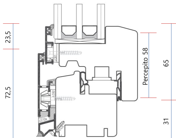
Traverso inferiore finestra
