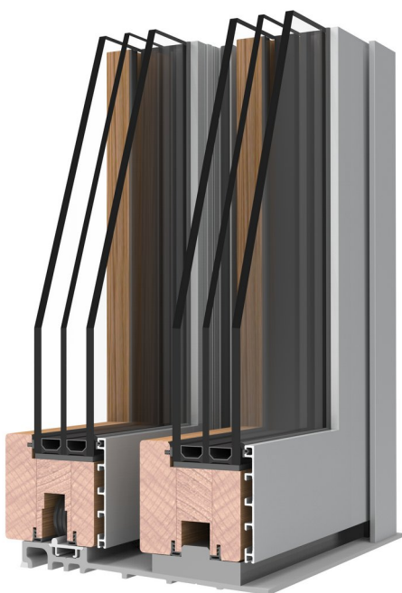
MODELLO SIMMETRICO
