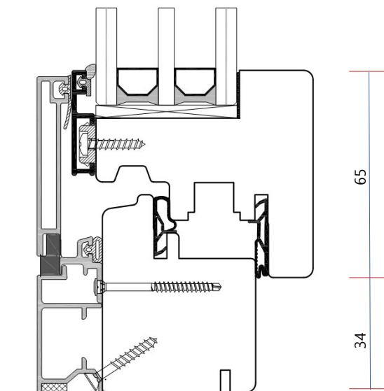
Traverso inf. Finestra
