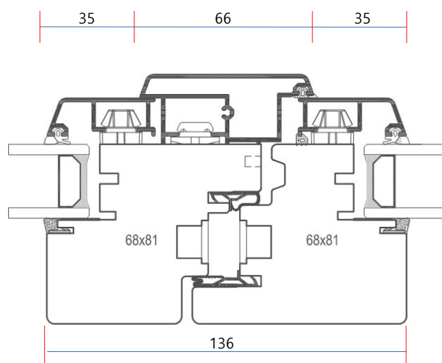
Nodo centrale doppio battente
