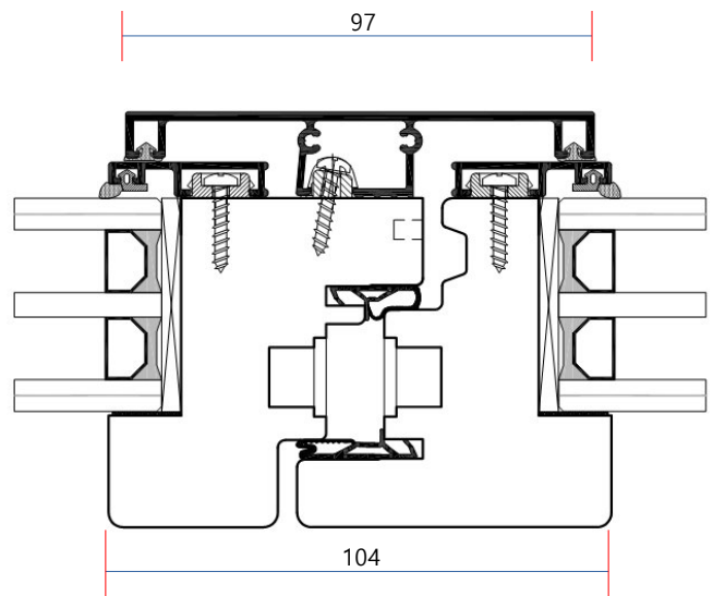
Nodo centrale doppio battente
