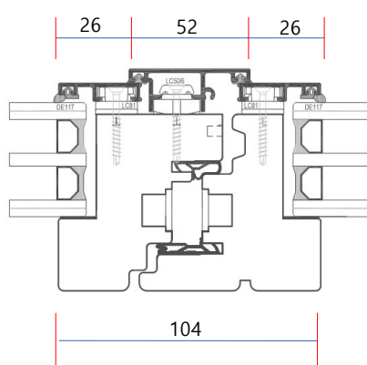
Nodo centrale 2 batt.
