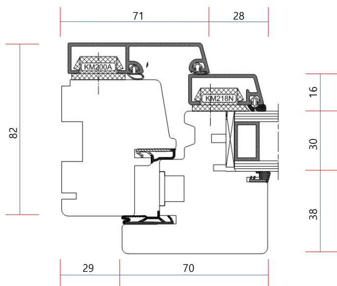
Telaio Fin/Pfin.
